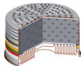
Dräger X-plore® Rd90 Filter: Schnittzeichnung
